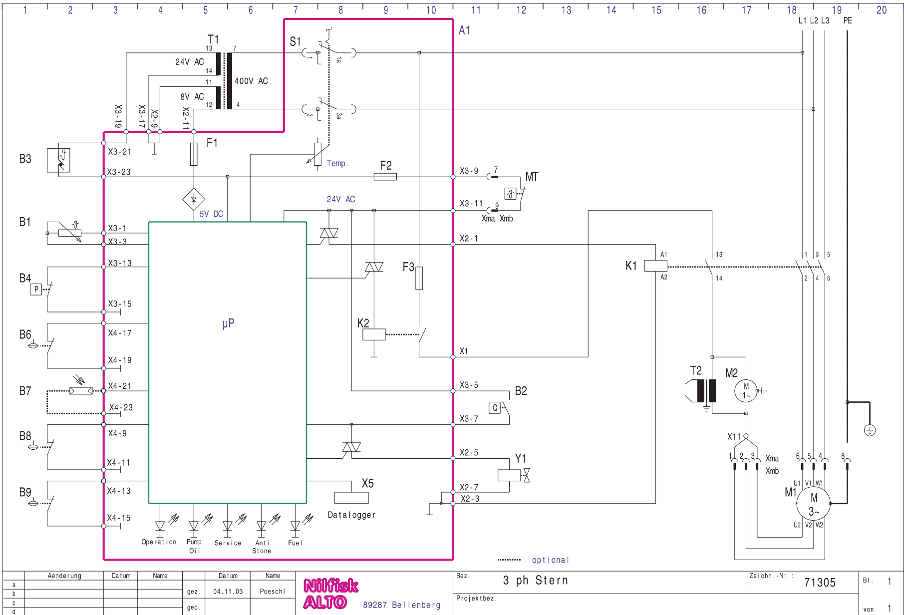
Fig. H.1: Wiring diagram 3~ star
